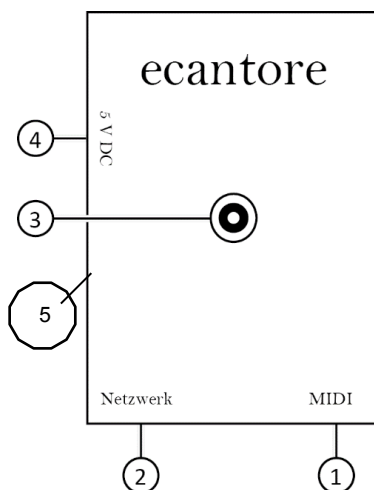
Abbildung 3 Schnittstellen der Orgelsteuerung
