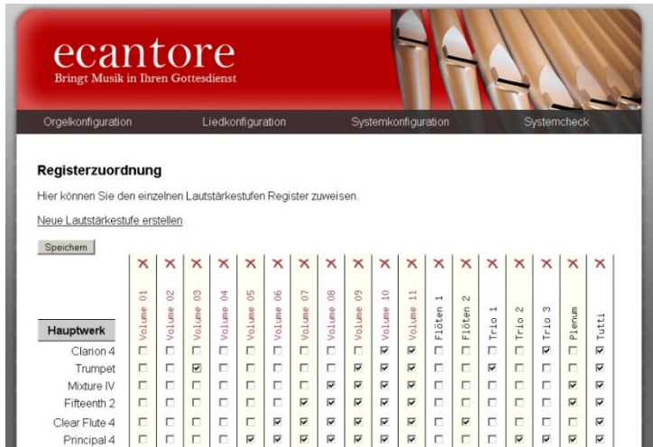
Abbildung 5 Registerzuordnung
