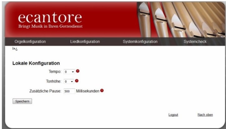
Abbildung 7 Globale Einstellungen
